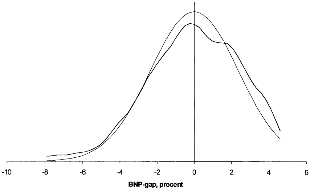
Figur 3: BNP-gapets fördelning
